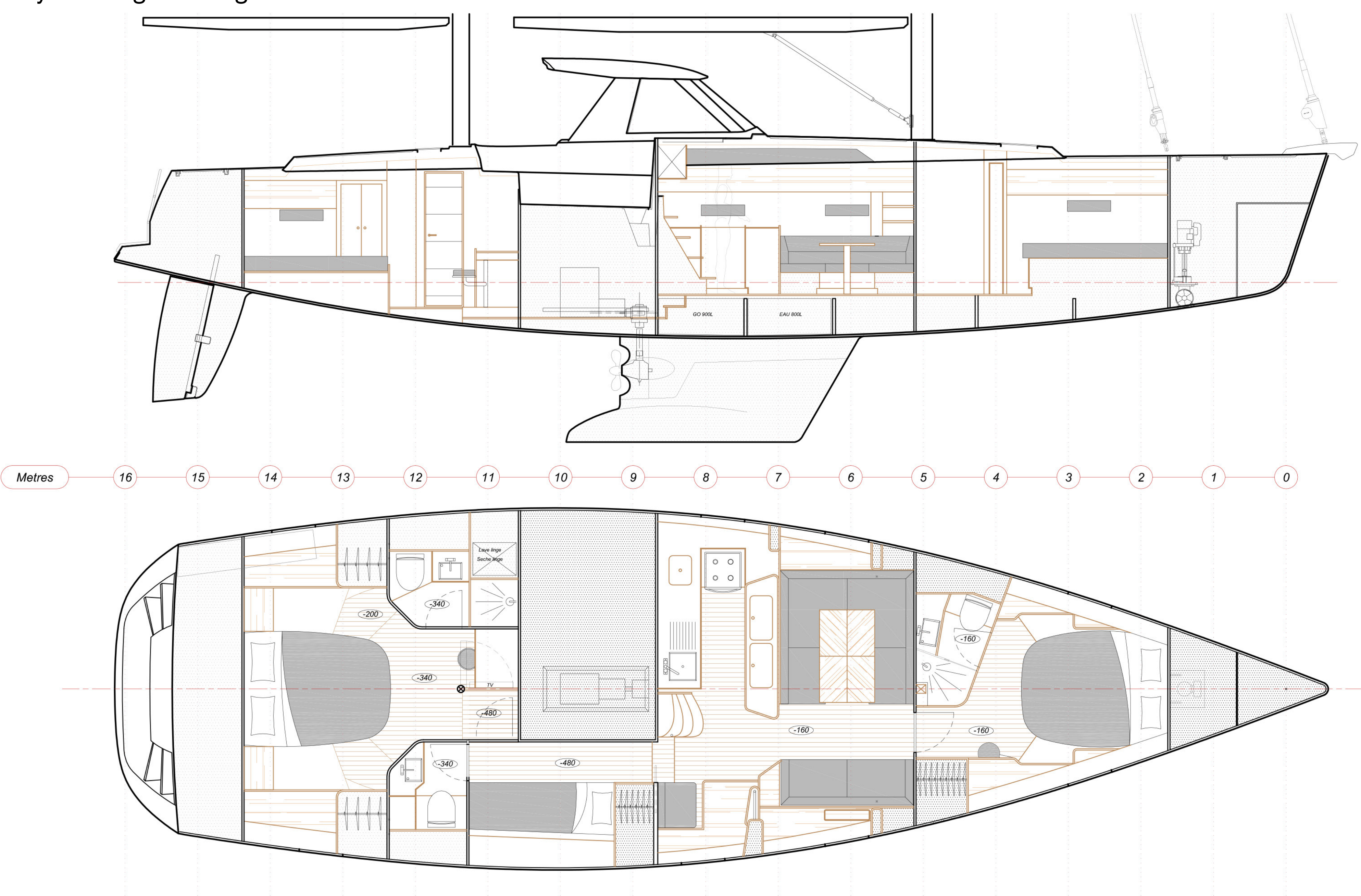
Layout mit großer Eignerkabine
